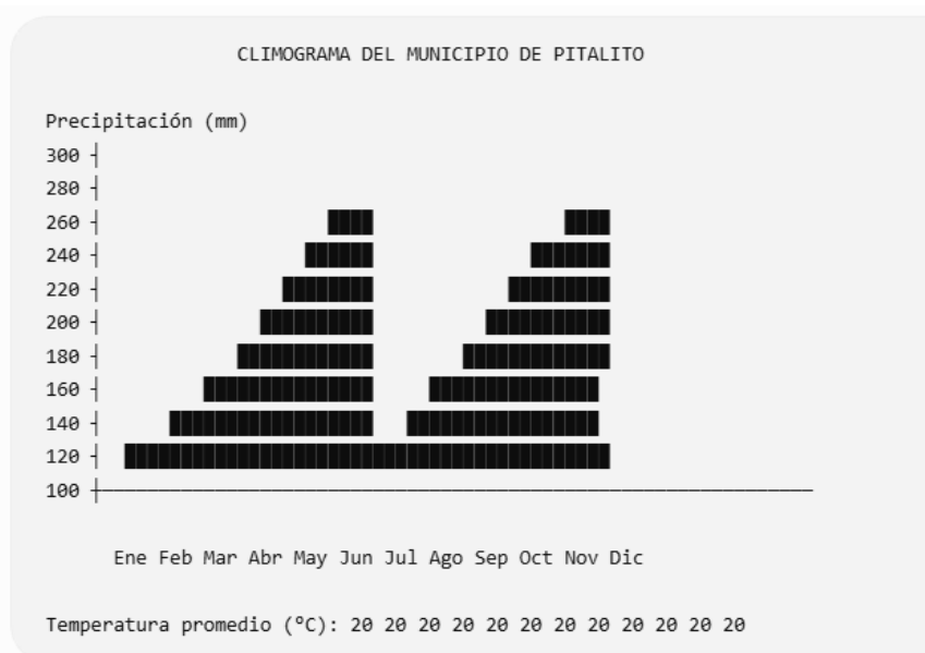
Figura 5. Comportamiento general de la precipitación y la temperatura en el municipio de Pitalito.
